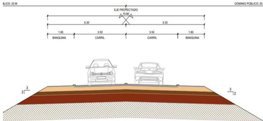
Figura N° 3. Sección tipo Variante Ypacaraí
