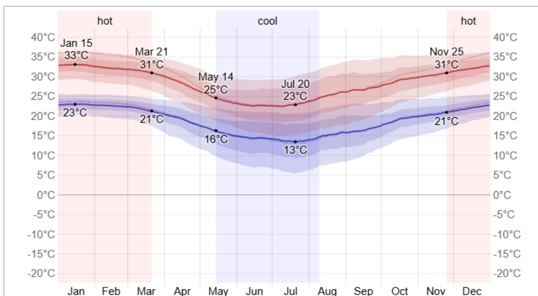
Figura N° 13. Datos históricos de temperatura en 2024 en el Aeropuerto Internacional de Asunción Silvio Pettirossi
