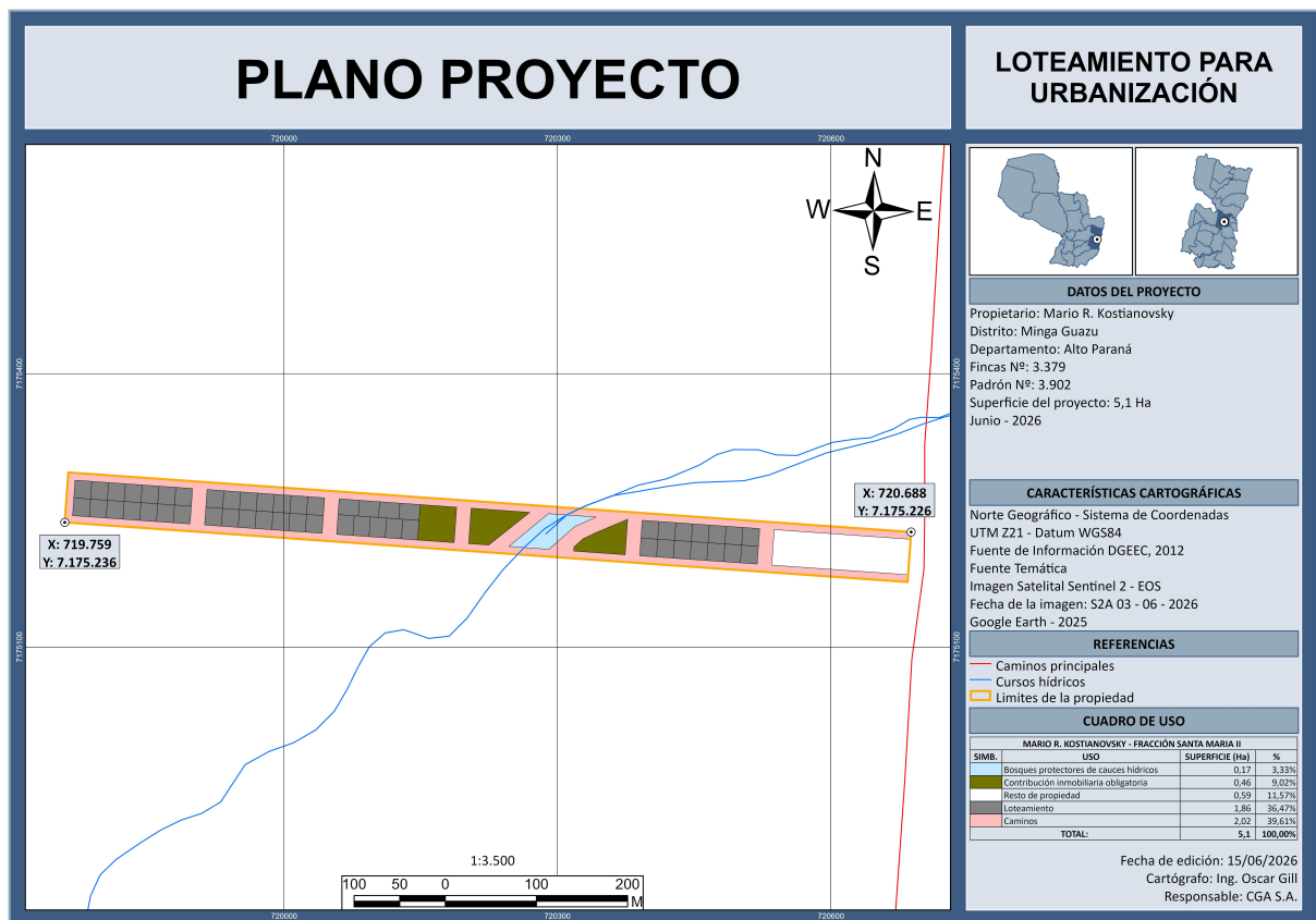
Imagen 4 Plano proyecto
