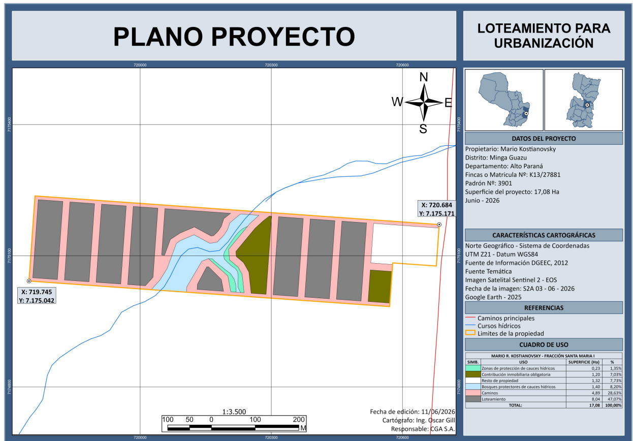
Imagen 4 Plano proyecto
