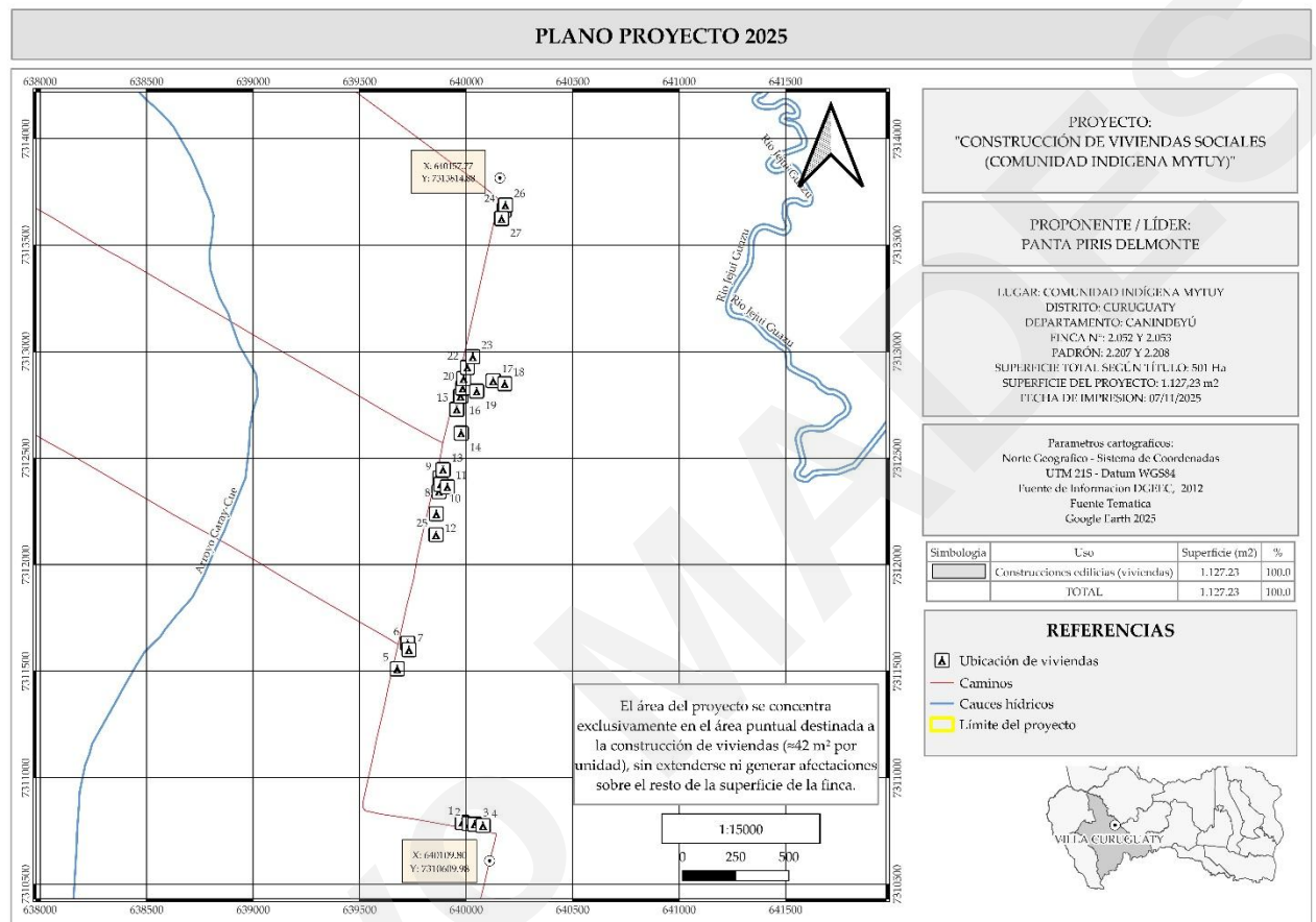
Imagen 3 Plano proyecto
