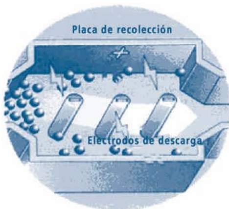
■ Figura 2. Principio del precipitador electrostático
