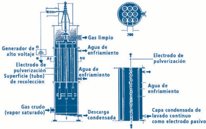
■ Figura 3. Precipitador electrostático por condensación
