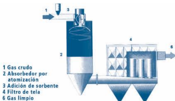
■ Figura 5. Adsorción/depuración con secado por atomización
