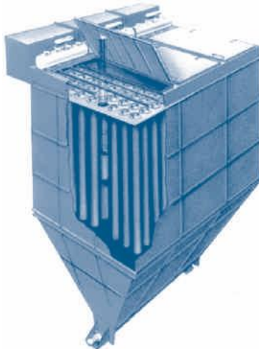
■ Figura 4. Esquema de un filtro de tela
