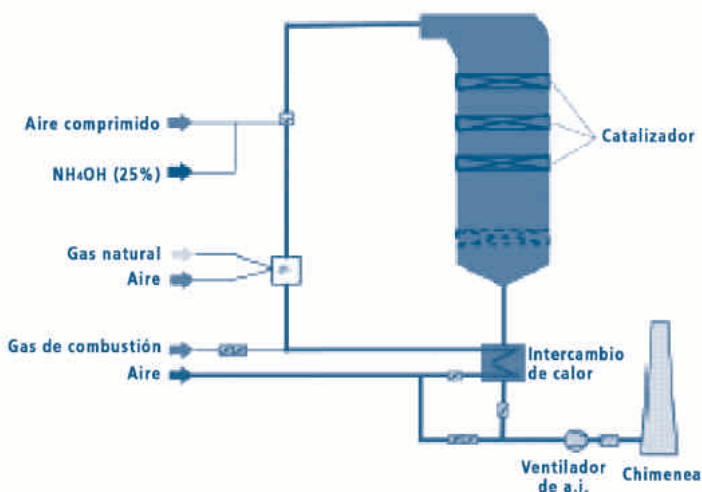
■ Figura 6. Reactor de reducción catalítica selectiva de alta temperatura para eliminar simultáneamente \text{NO}_x y PCDD/PCDF
