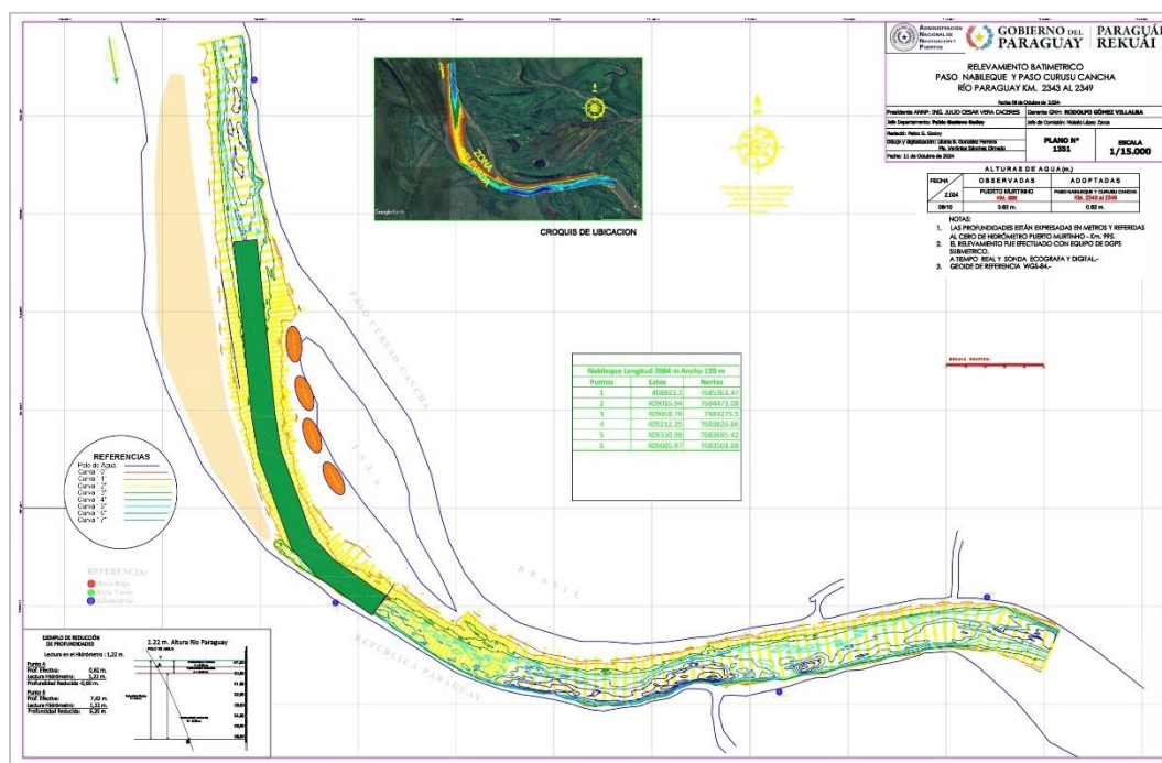
Figura N° 3. Área de dragado (polígono verde) y áreas de vaciado (polígonos naranjas). Fuente: El proponente.
