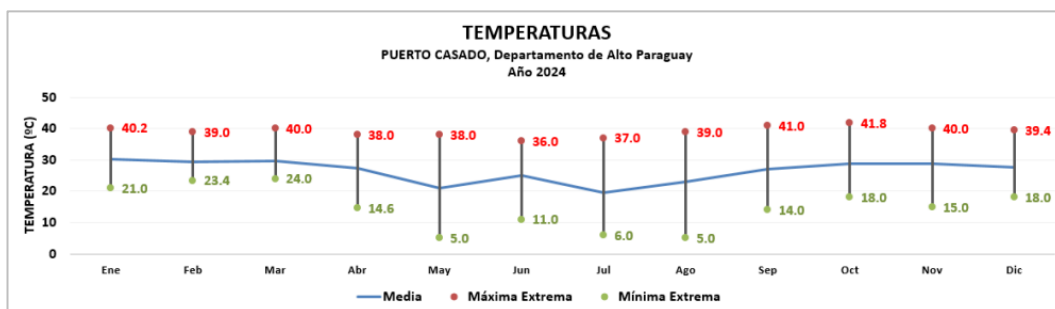
Figura N° 10. Temperatura media mensual y valores extremos mensuales de la máxima y mínima
