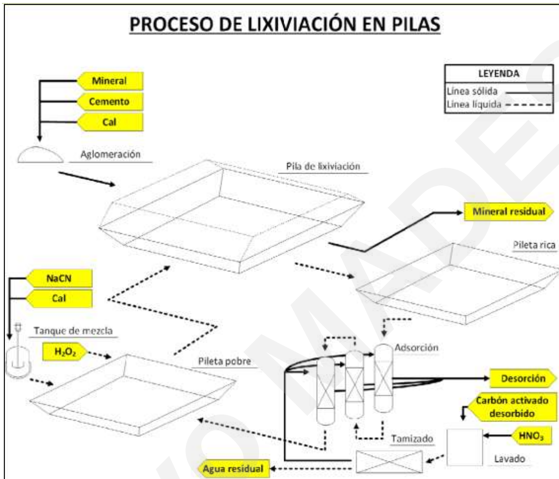
Figura 1. Proceso de lixiviación en pilas.
