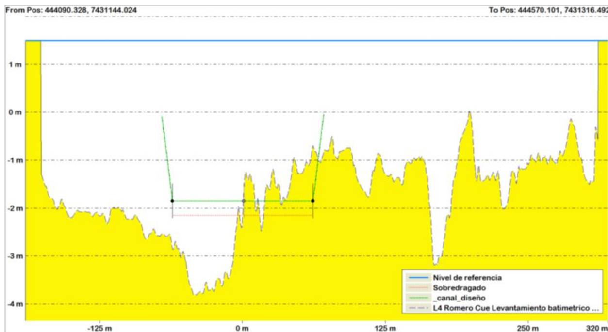
Figura 6. Sección transversal del Paso Romero Cué
