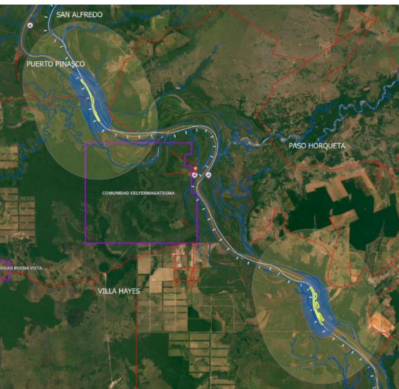
Figura 10. Ubicación de zona de dragado y zona de vertido/vaciado
