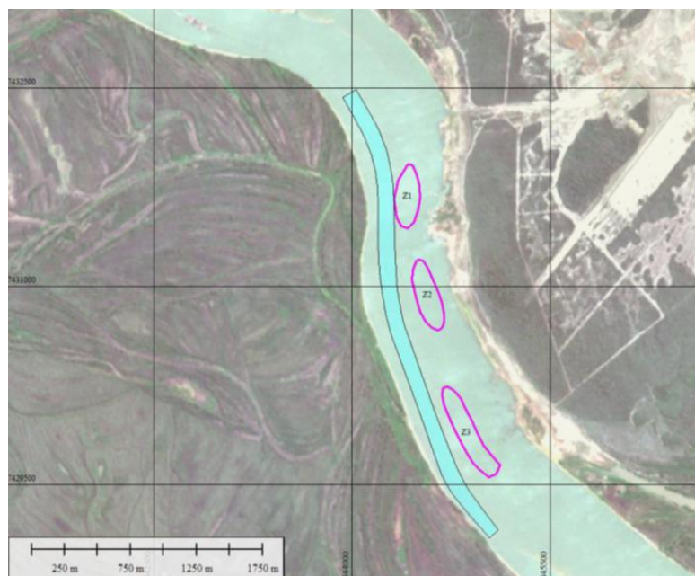
Figura 5. Polígono del dragado (celeste) en el Paso Romero Cué
