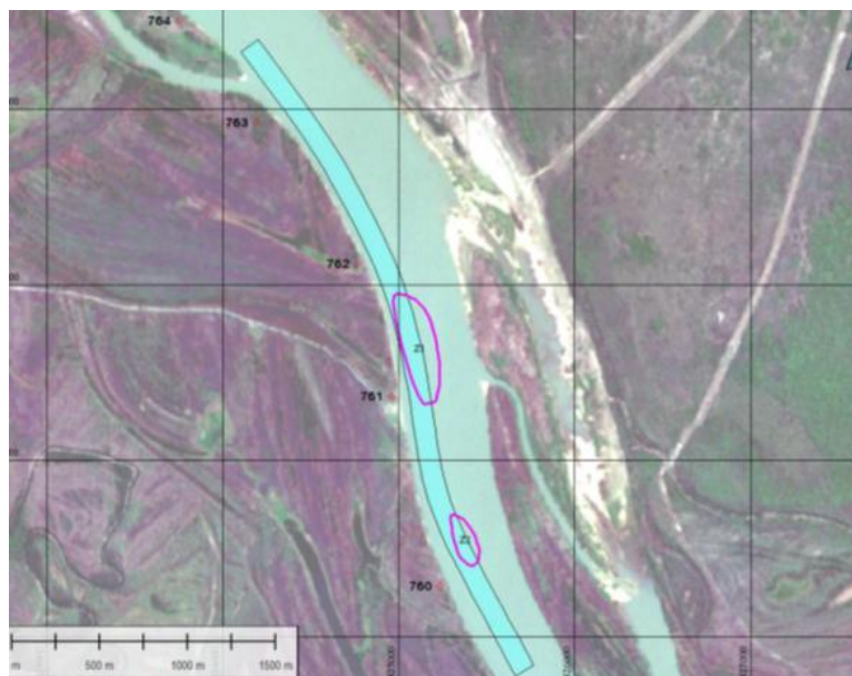
Figura 3. Polígono del dragado (celeste) en el Paso San Juan
