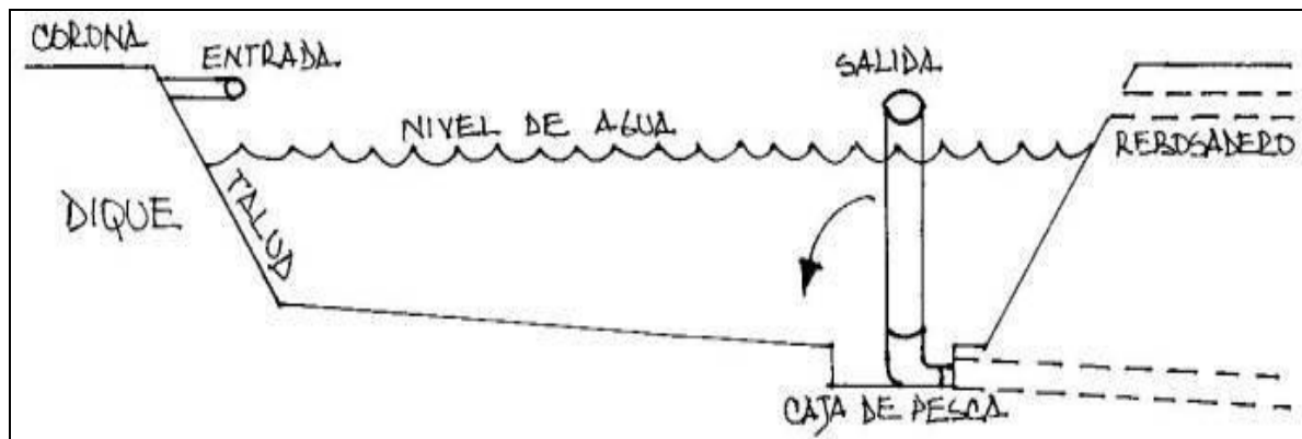
Figura 1. Partes que conforman un estanque en tierra.
