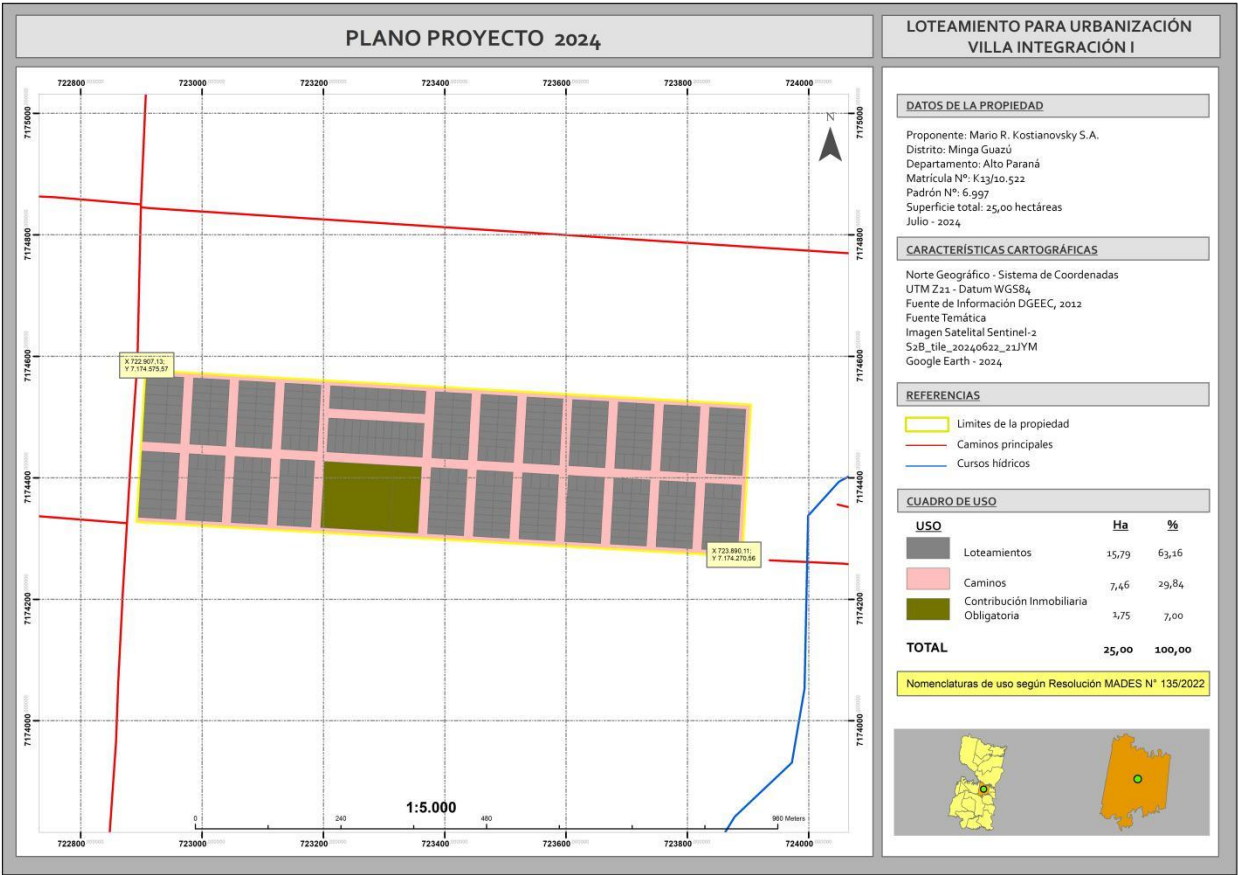
Imagen 4 Plano proyecto
