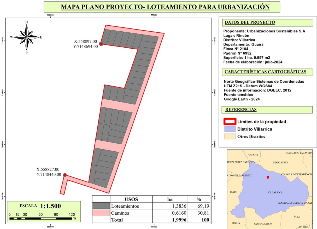
Imagen 4 Plano del proyecto
