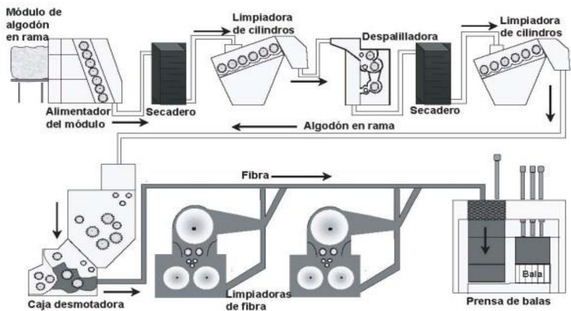
Figura 3 Flujograma estándar del proceso del desmotado de algodón
