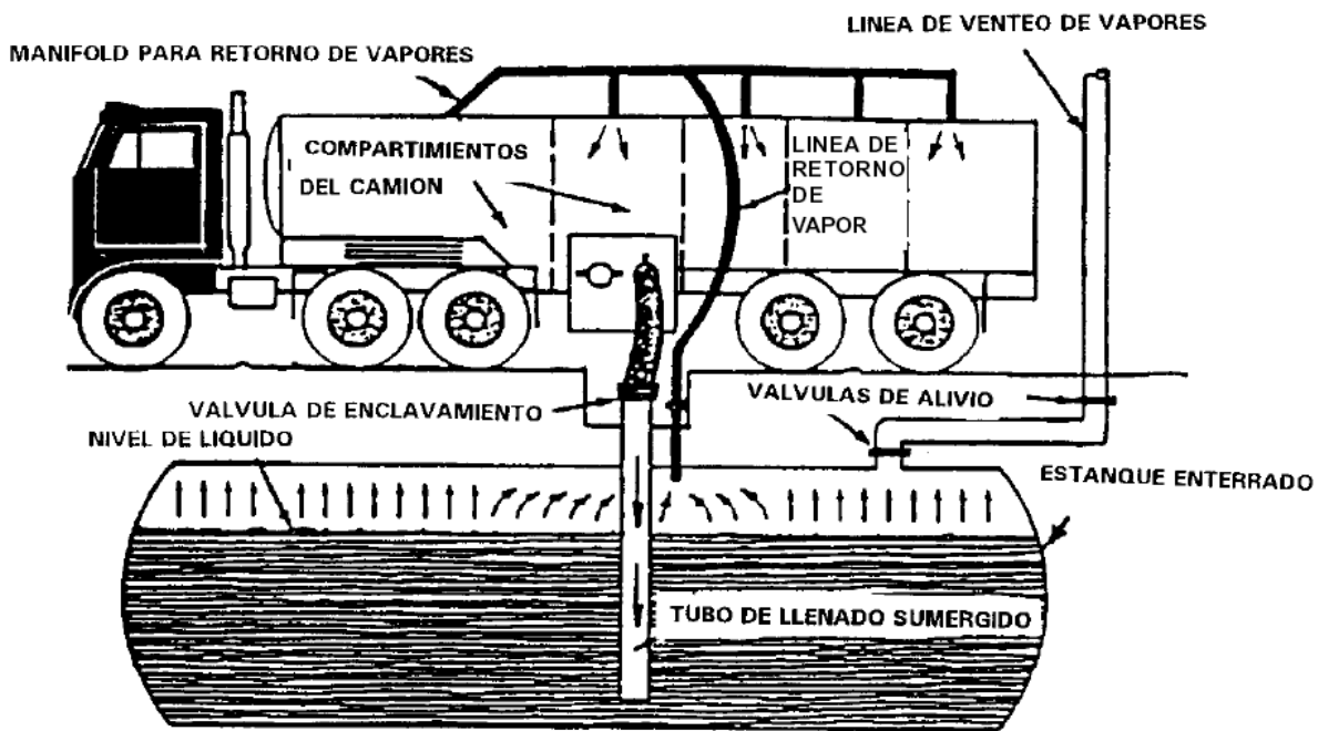
Figura 1: Descargue de combustible en la Estación de Servicio con traspaso de vapores.
